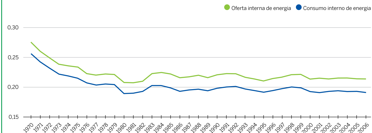
GRÁFICO 5 • Oferta interna e consumo final de energia por unidade de PIB – Brasil, 1970 a 2006 (tep - tonelada equivalente de petróleo/mil US$)
