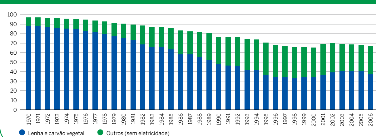
GRÁFICO 12 • Participação da preparação de alimentos no uso residencial de energia – Brasil, 1970 a 2006
